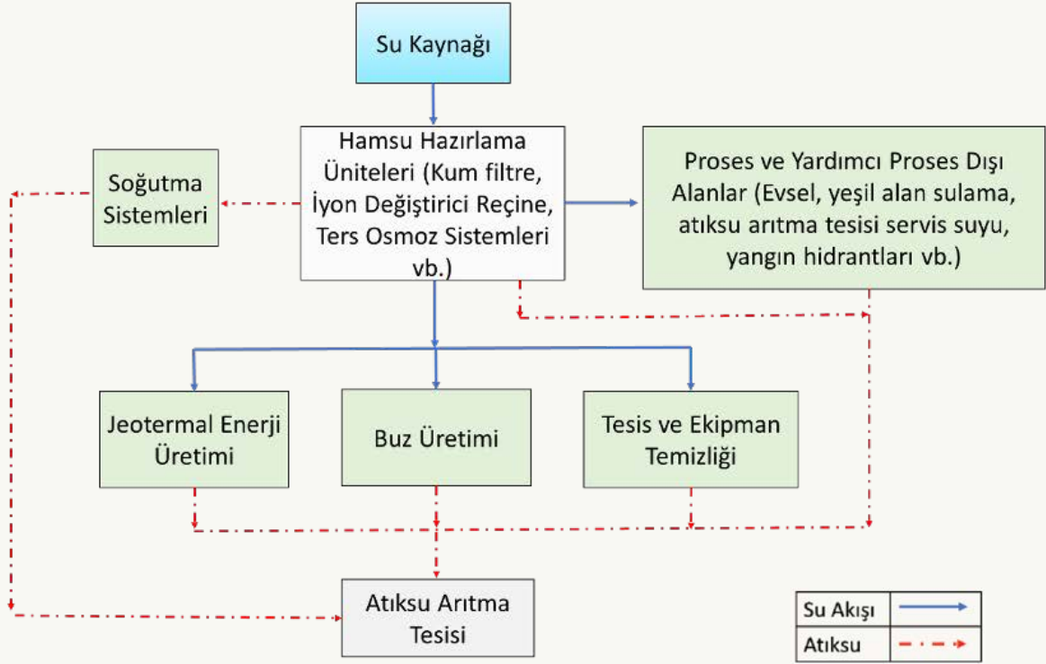
Buhar ve İklimlendirme Temini Sektörü Su Akım Şeması
