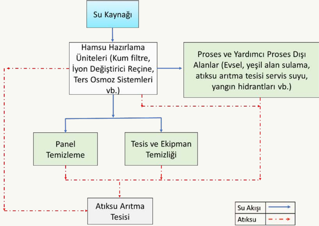
Elektrik Enerjisi Üretimi Sektörü Su Akım Şeması
