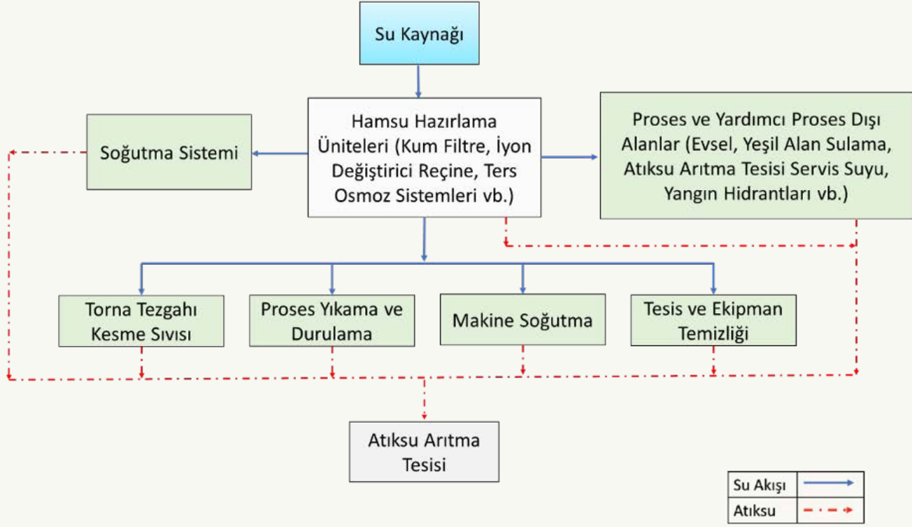
Tekstil, Giyim Eşyası ve Deri Üretiminde Kullanılan Makinelerin İmalatı Sektörü Su Akım Şeması
