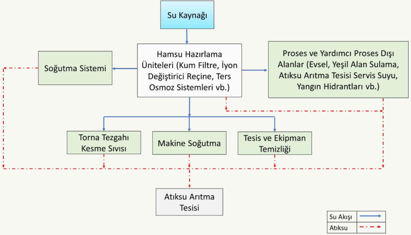
Kaldırma ve Taşıma Ekipmanları İmalatı Sektörü Su Akım Şeması
