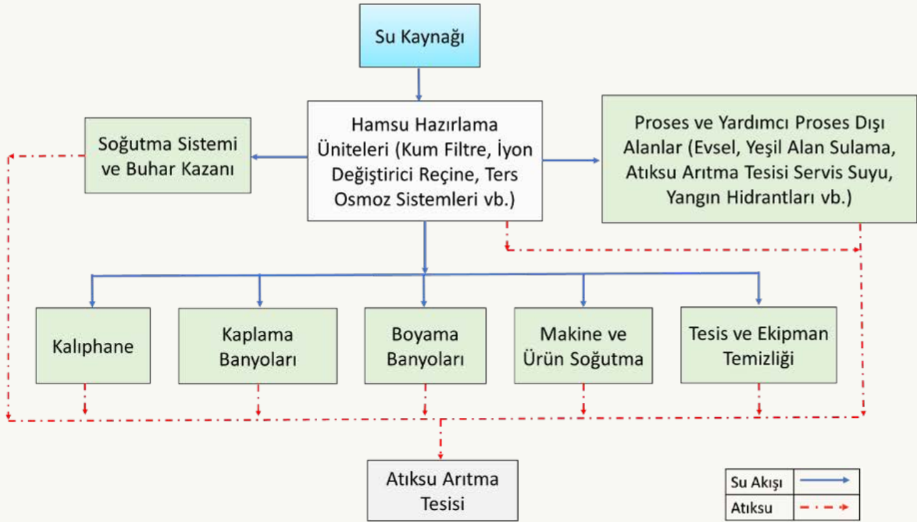
Elektrikli Ev Aletlerinin İmalatı Sektörü Su Akım Şeması
