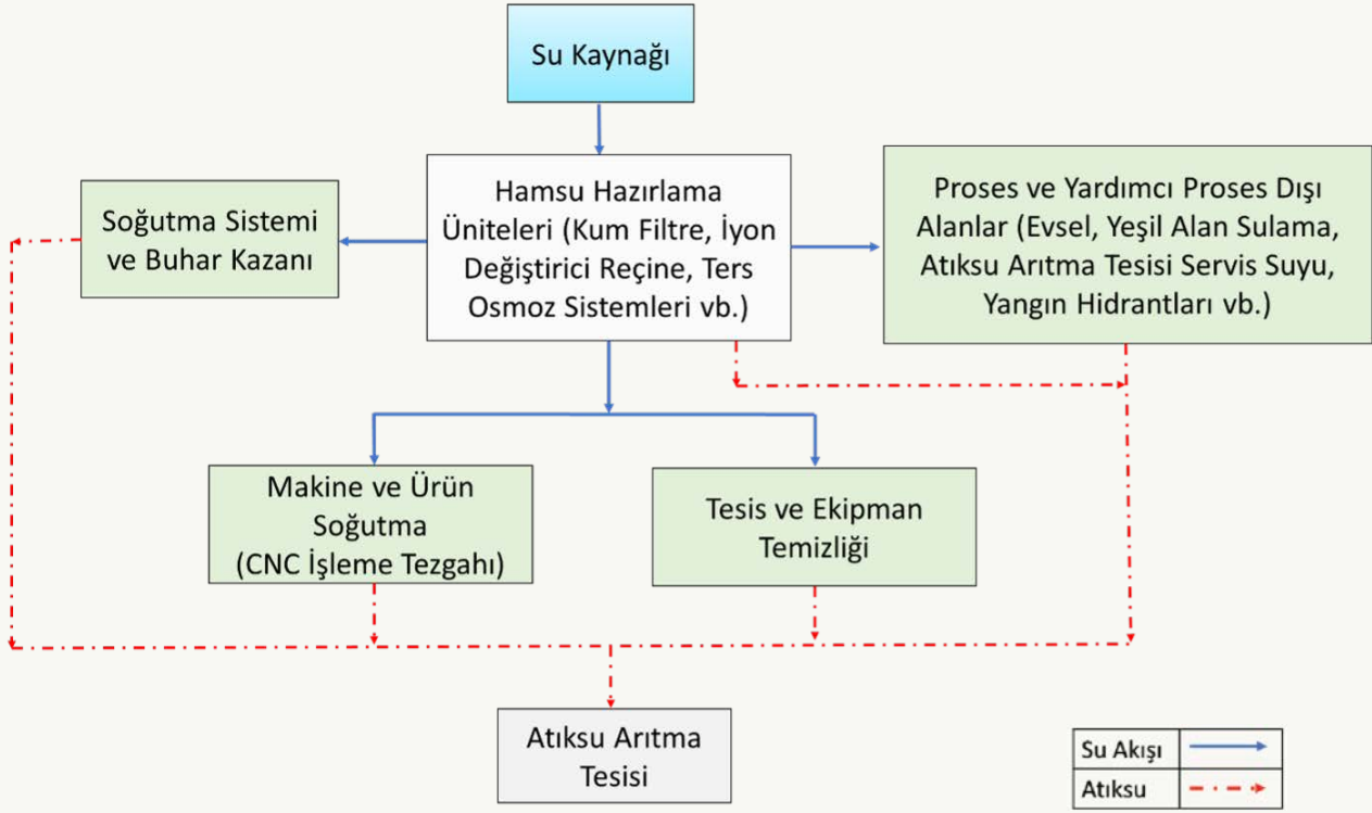
Elektrikli Aydınlatma Ekipmanlarının İmalatı Sektörü Su Akım Şeması
