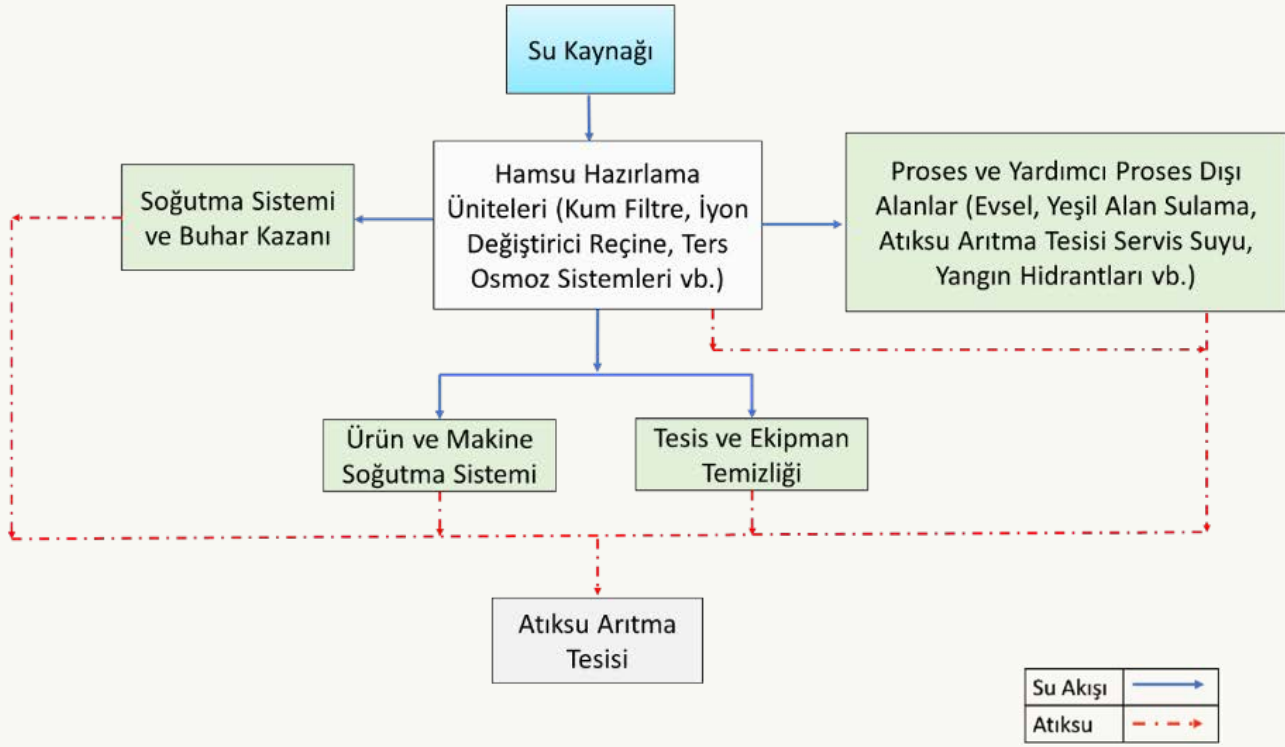
Diğer Elektronik ve Elektrik Telleri ve Kablolarının İmalatı Sektörü Su Akım Şeması
