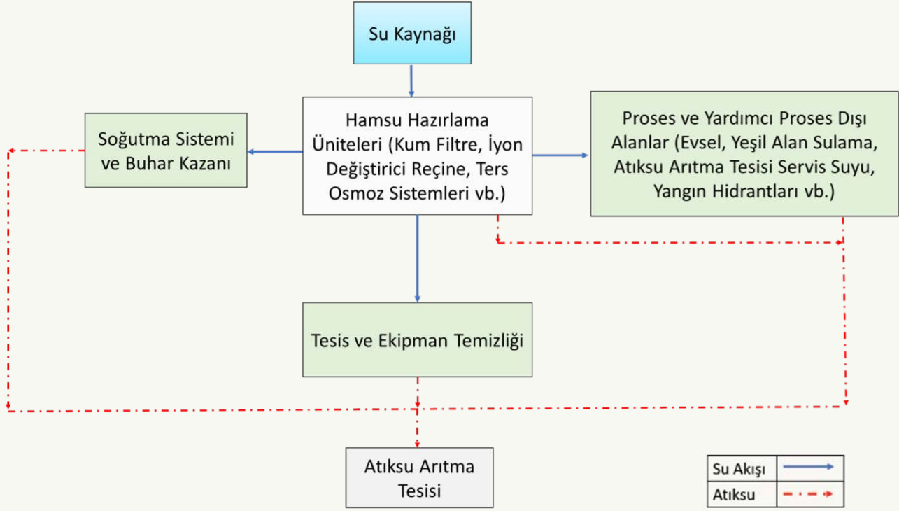
Fiber Optik Kabloların İmalatı Sektörü Su Akım Şeması
