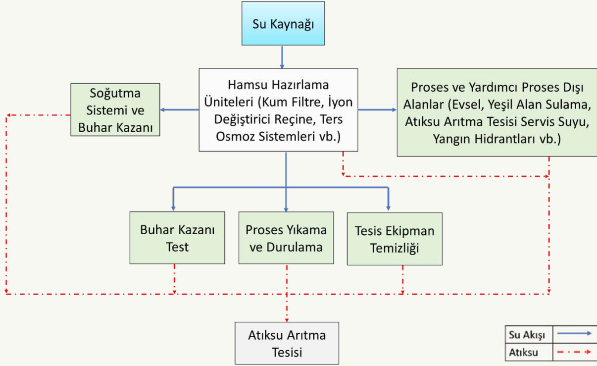
Buhar Jeneratörü İmalatı, Merkezi Isıtma Sıcak Su Kazanları (Boylarları) Hariç, Sektör Su Akım Şeması
