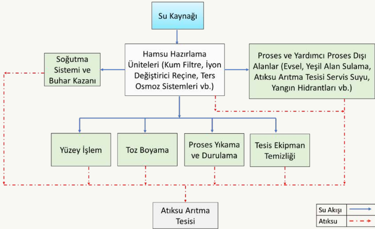
Merkezi Isıtma Radyatörleri (Elektrikli Radyatörler Hariç) ve Sıcak Su Kazanları (Boyerleri) İmalatı Sektörü Su Akım Şeması
