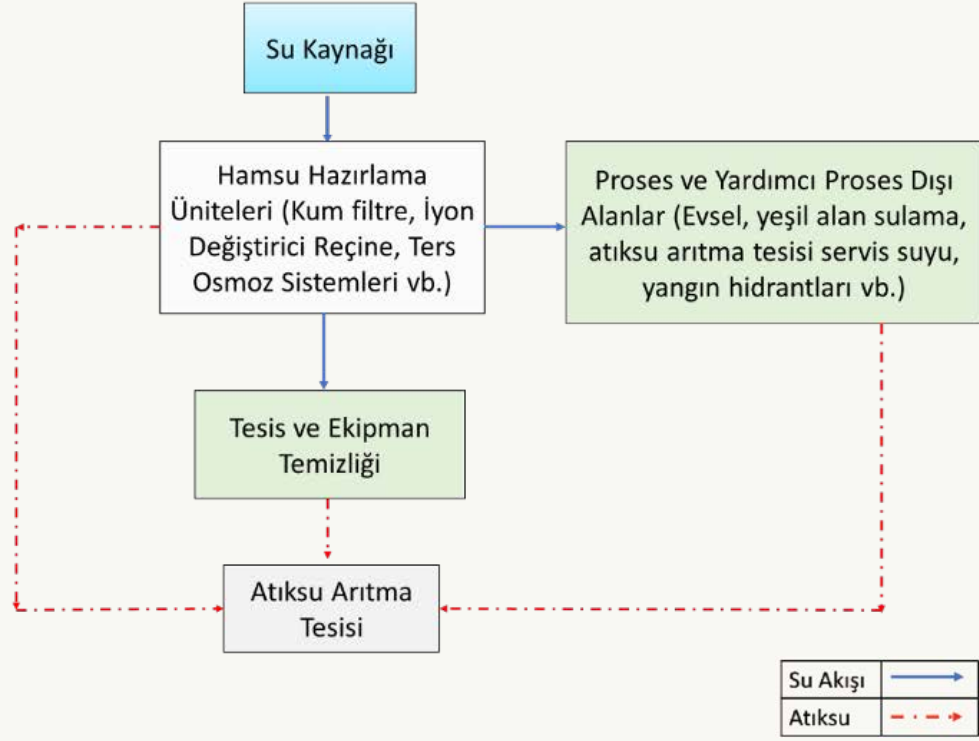
Metalden Kapı ve Pencere İmalatı Sektörü Su Akım Şeması
