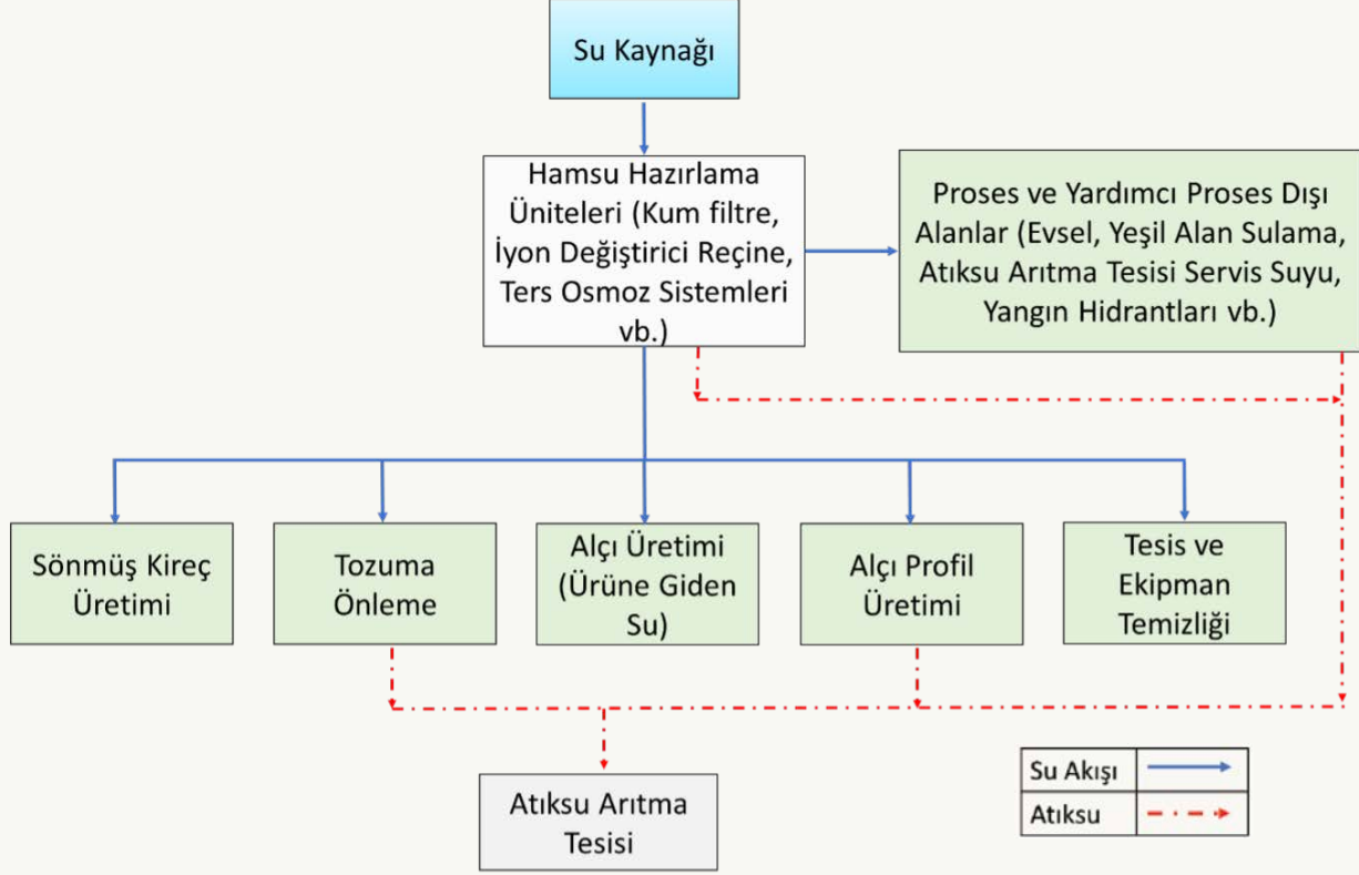
Kireç ve Alçı İmalatı Sektörü Su Akım Şeması
