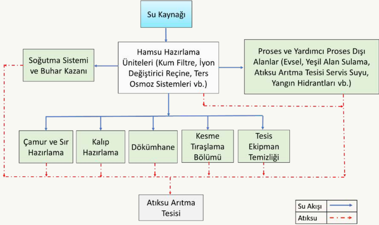
Seramik Sıhhi Ürünlerin İmalatı Sektörü Su Akım Şeması
