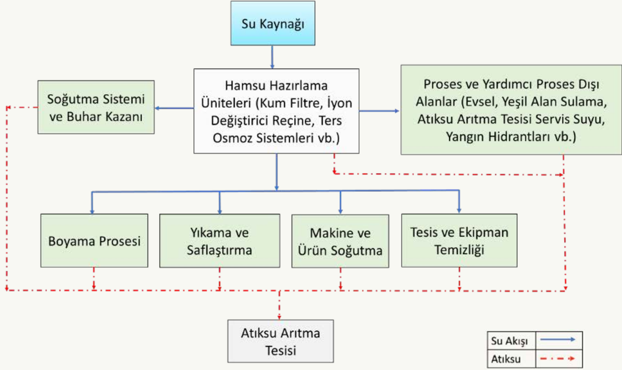
Çukur Cam İmalatı Sektörü Su Akım Şeması
