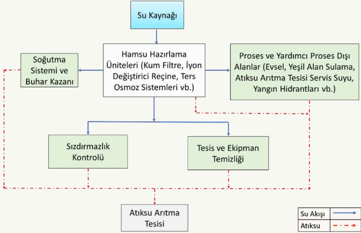
Plastik İnşaat Malzemesi İmalatı Sektörü Su Akım Şeması
