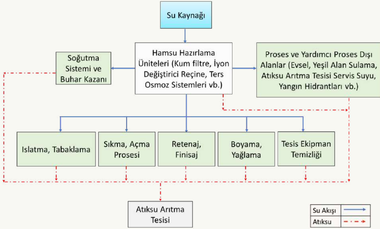
Derinin Tabaklanması ve İşlenmesi; Kürkün İşlenmesi ve Boyanması Su Akım Şeması
