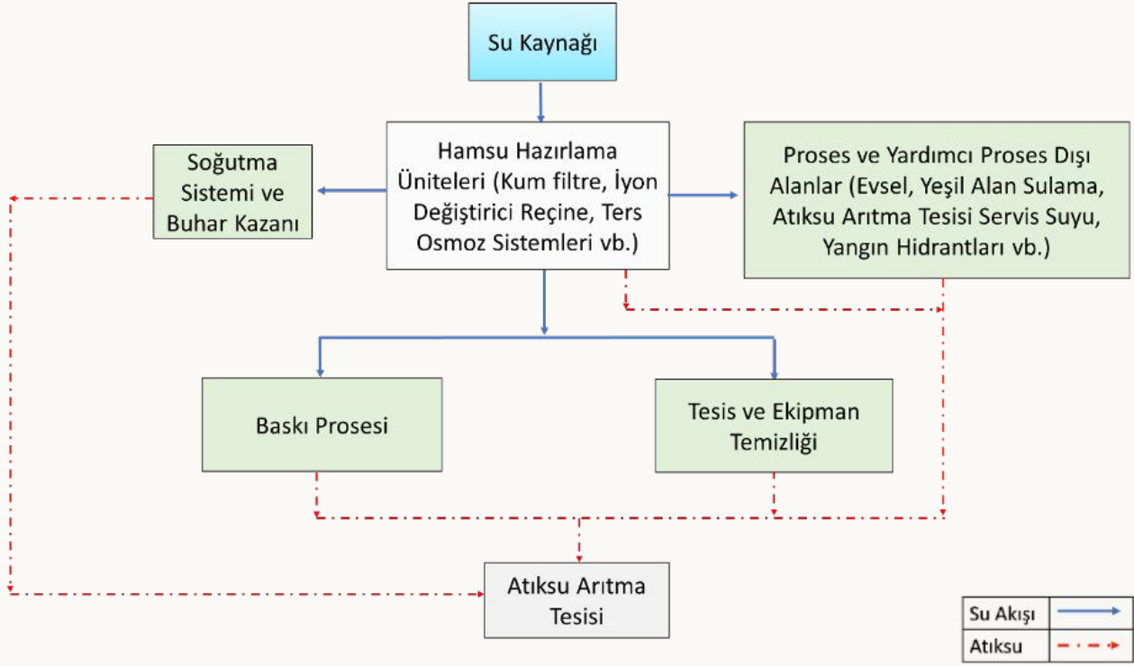
Başka Yerde Sınıflandırılmamış Diğer Tekstillerin İmalatı Sektörü Su Akım Şeması
