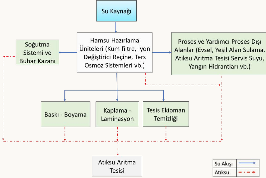
Halı ve Kilim İmalatı Sektörü Su Akım Şeması
