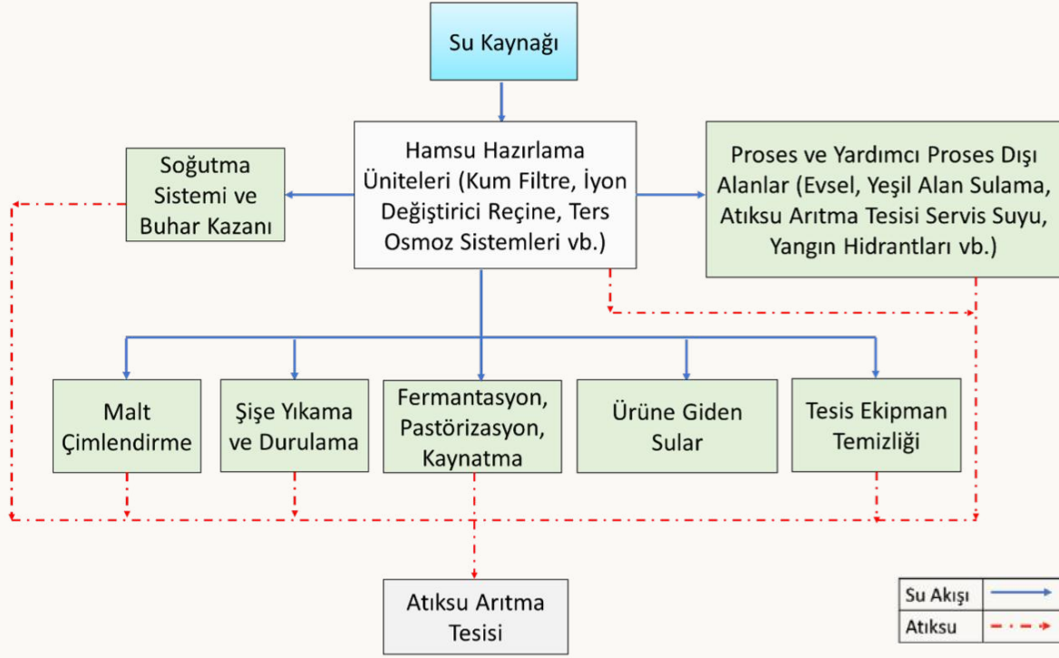
Bira İmalatı Su Akım Şeması
