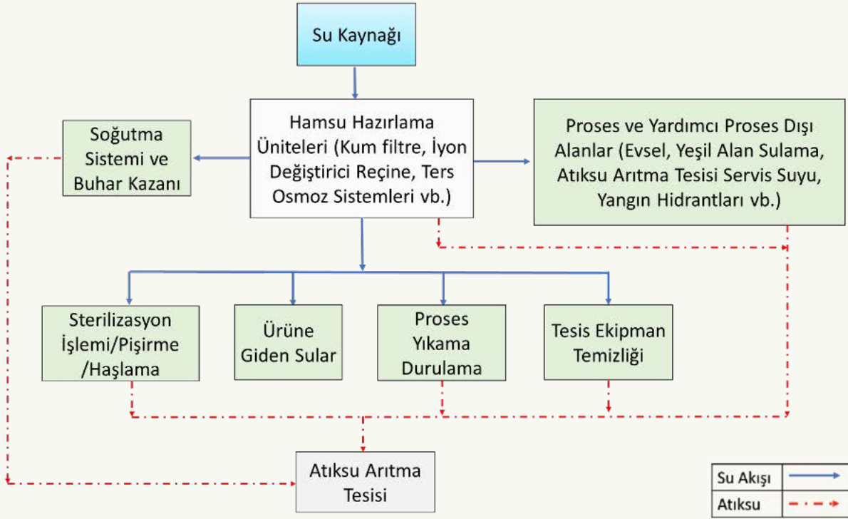
Hazır Yemeklerin İmalatı Sektörü Su Akım Şeması
