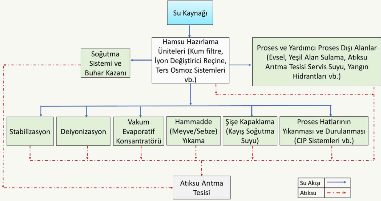
Sebze ve Meyve Suyu İmalatı Sektörü Su Akım Şeması
