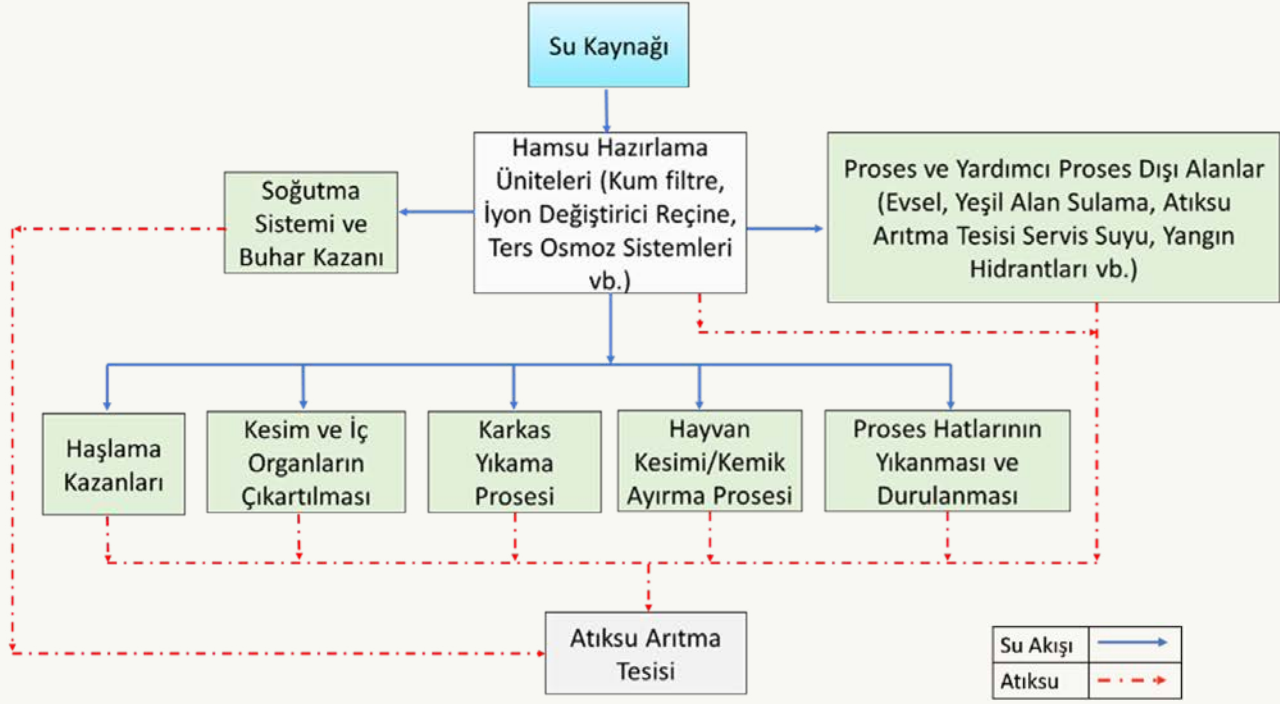
Etin İşlenmesi ve Saklanması Sektörü Su Akım Şeması
