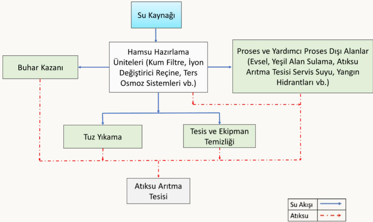
Tuz Çıkarımı Sektörü Su Akım Şeması
