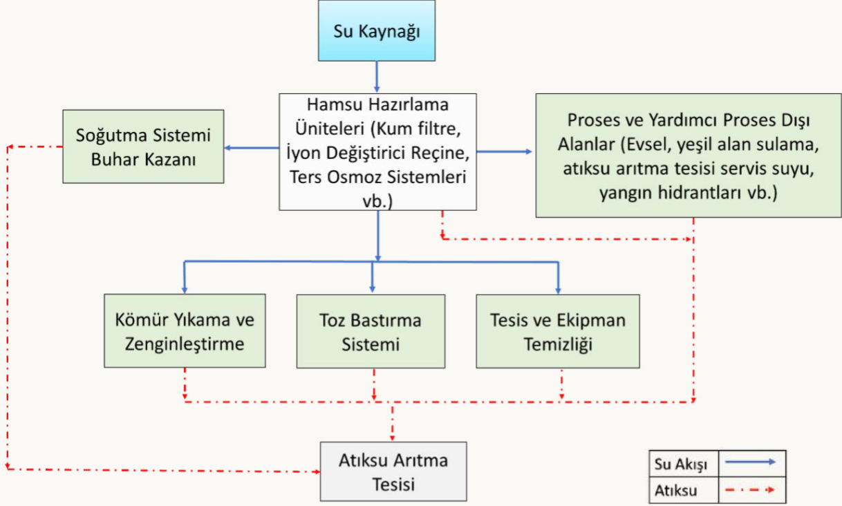
Linyit Madenciliği Sektörü Su Akım Şeması
