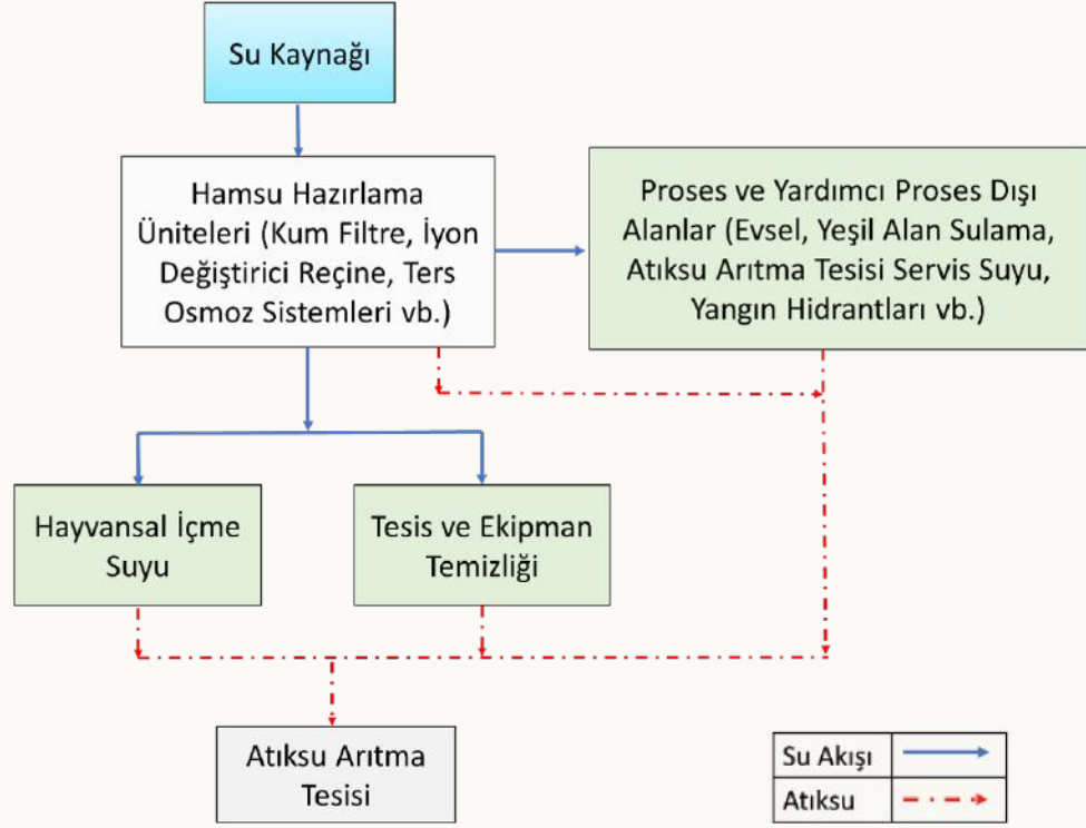
Koyun ve Keçi Yetiştiriciliği Sektörü Su Akım Şeması
